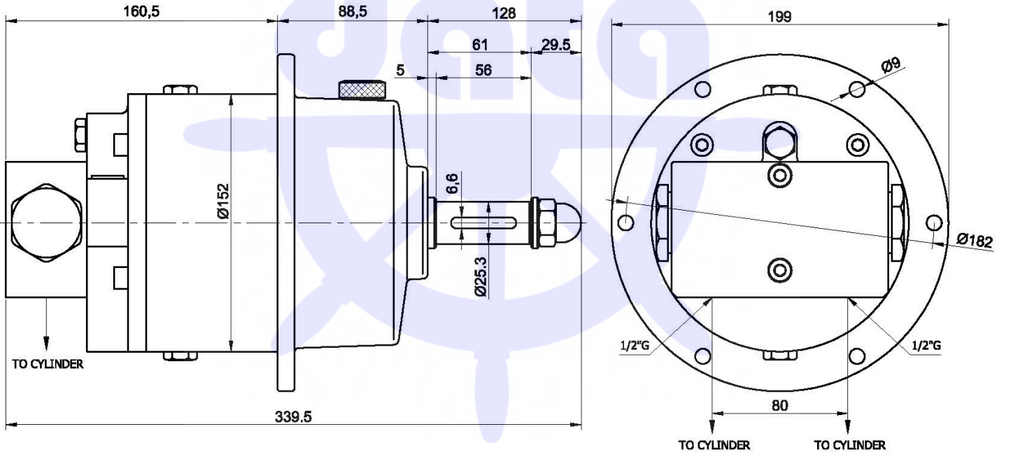
DP 63K - DP 75K - DP 88K
