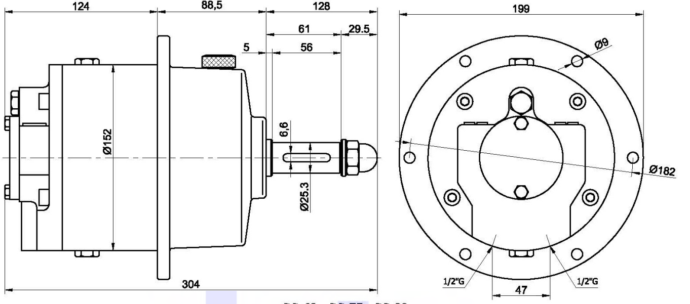
DP 63 - DP 75 - DP 88
