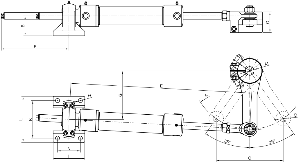
Şekil-1 (drw.1)
